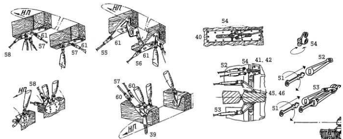
Узлы крепления центроплана и крыльев
